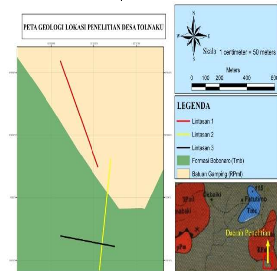
Gambar 3. Peta geologi lokasi penelitian
