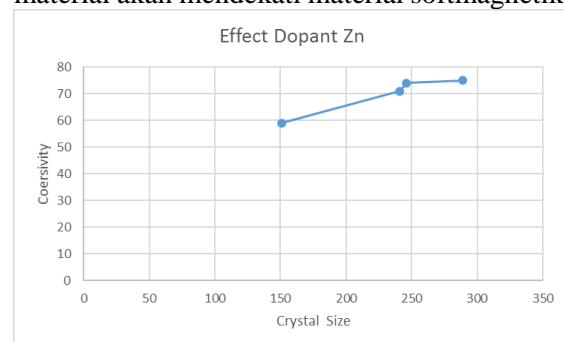
Gambar 5. Hubungan nilai koersivitas dengan ukuran kristal
