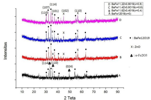
Gambar 1. Pola XRD dari 4 sampel BaFe_{12}O_{19}
