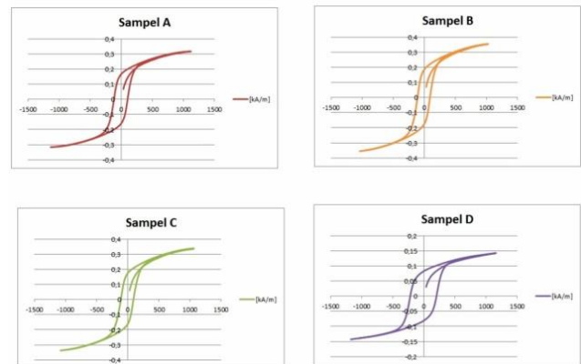
Gambar 3. Kurva hysteresis Barium Heksaferit yang didoping ZnO
