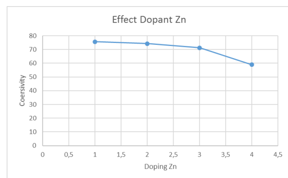
Gambar 4. Hubungan doping Zn dengan nilai koersivitas
