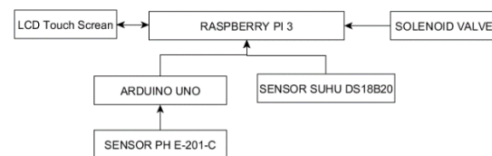
Gambar 10 Diagram blok sistem otomatisasi penyesuaian kadar pH
