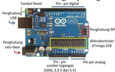
Gambar 6 Bagian-bagian penting di arduino
