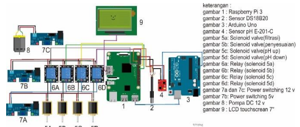
Gambar 15 perancangan keseluruhan sistem
