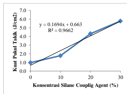
Gambar 4. Grafik Pengaruh Perlakuan Silane Coupling Agent Terhadap Kuat Pukul Takik Komposit
