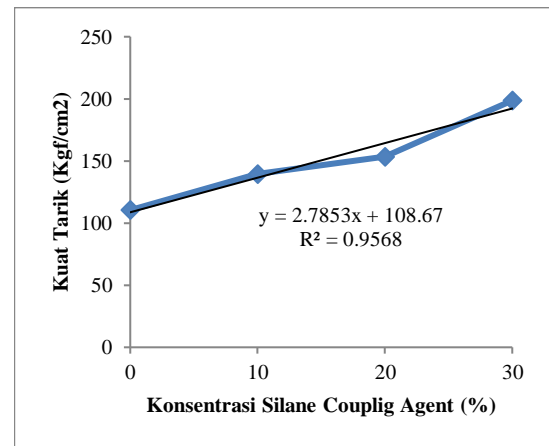
Gambar 3. Grafik Pengaruh Perlakuan Silane Coupling Agent Terhadap Kuat Tarik Komposit
