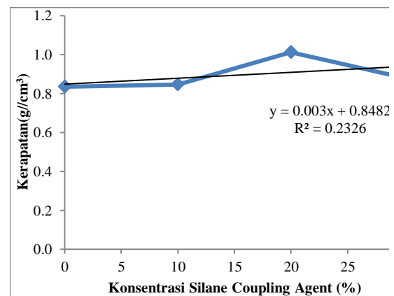
Gambar 1. Grafik Pengaruh Perlakuan Silane Coupling Agent Terhadap Kerapatan Komposit
