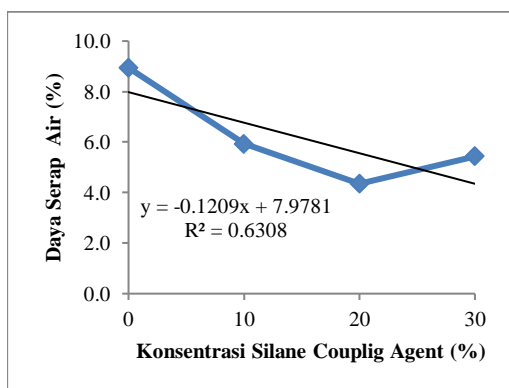
Gambar 2. Grafik Pengaruh Perlakuan Silane Coupling Agent Terhadap Daya Serap Air Komposit
