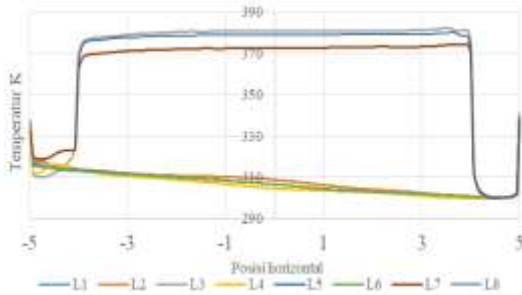
Gambar 8. Distribusi temperatur dengan beban terhadap posisi horizontal (garis virtual pada jam 13:00 dengan kecepatan 0,5 m/s.
