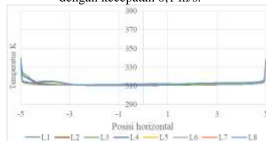
Gambar 18. Distribusi temperatur tanpa beban terhadap posisi horizontal (garis virtual) pada jam 13:00 dengan kecepatan 1,36 m/s.
