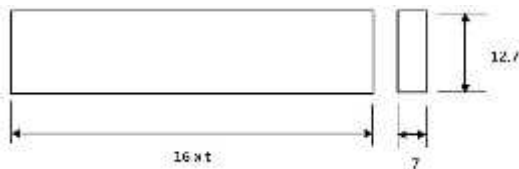
Gambar 3. Dimensi spesimen uji bending ASTM D790.
