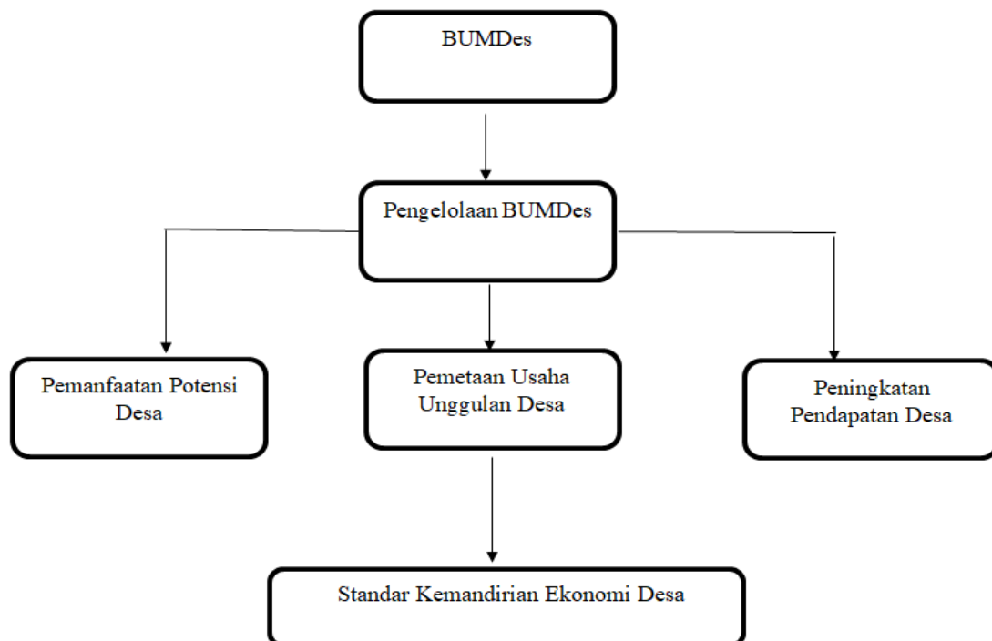
Gambar 1. Kerangka Berpikir
