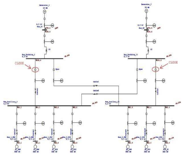
Gambar 3 Simulasi load flow analysis pada ETAP 12.6.0 kondisi Pertama
