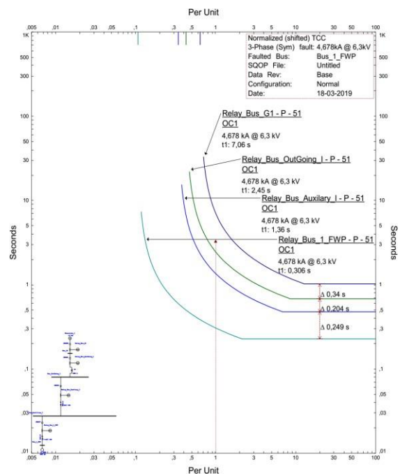
Gambar 4 Kurva Koordinasi Motor 1 FWP
