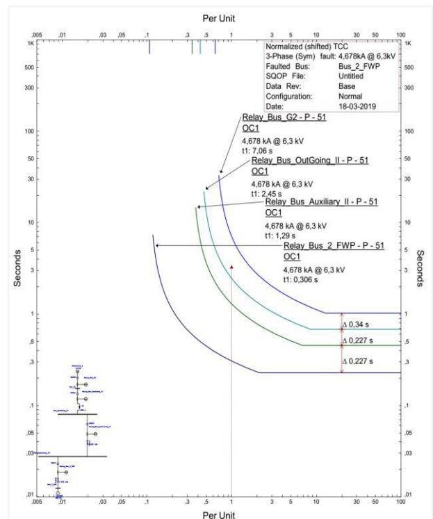
Gambar 6 Kurva Koordinasi Motor 2 FWP
