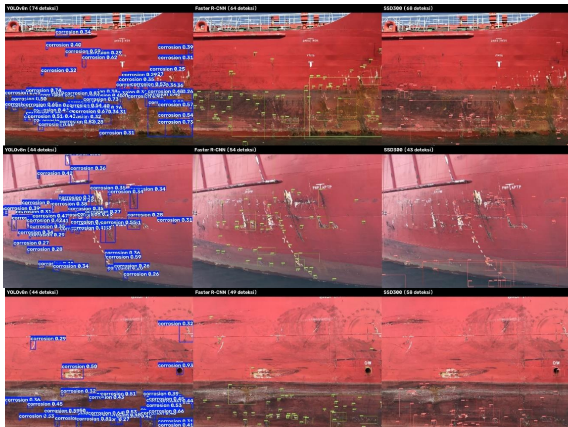
Gambar 1. Perbandingan hasil deteksi korosi lambung kapal pada citra uji HiRes_hull007 (atas), HiRes_hull017 (tengah), dan HiRes_hull024 (bawah). Kolom kiri: YOLOv8n (biru), kolom tengah: Faster R-CNN (hijau), kolom kanan: SSD300 (merah muda). Angka dalam kurung menunjukkan jumlah area korosi yang terdeteksi pada masing-masing model.
