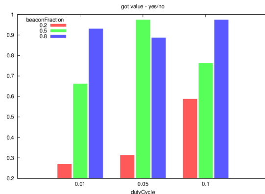
Gambar 3 Pengaruh Duty Cycle dan Beacon Fraction terhadap PDR
