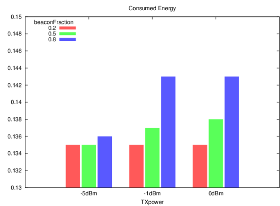
Gambar 7 Pengaruh Daya Transmisi terhadap Konsumsi Energi Jaringan
