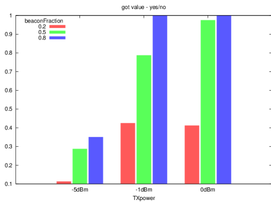
Gambar 4 Pengaruh Daya Transmisi terhadap PDR
