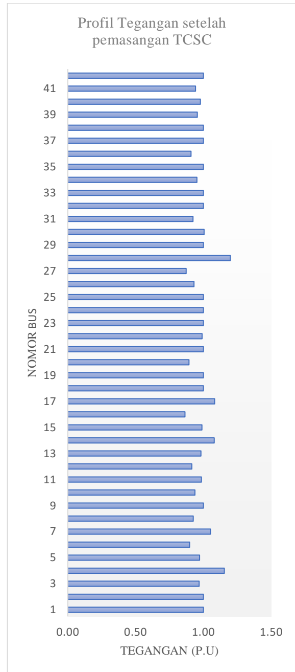
Gambar 6 Grafik Profil Tegangan Setelah Pemasangan TCSC
