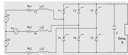
Gambar 1 Rangkaian penyearah terkendali 3 fasa gelombang penuh
